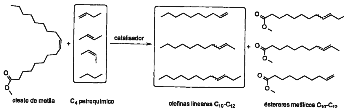
Figura 3: Esquema reacional para produção de olefinas C 10 -C 12 por metátese do oleato de metila e butenos de corte C 4 de craqueamento
